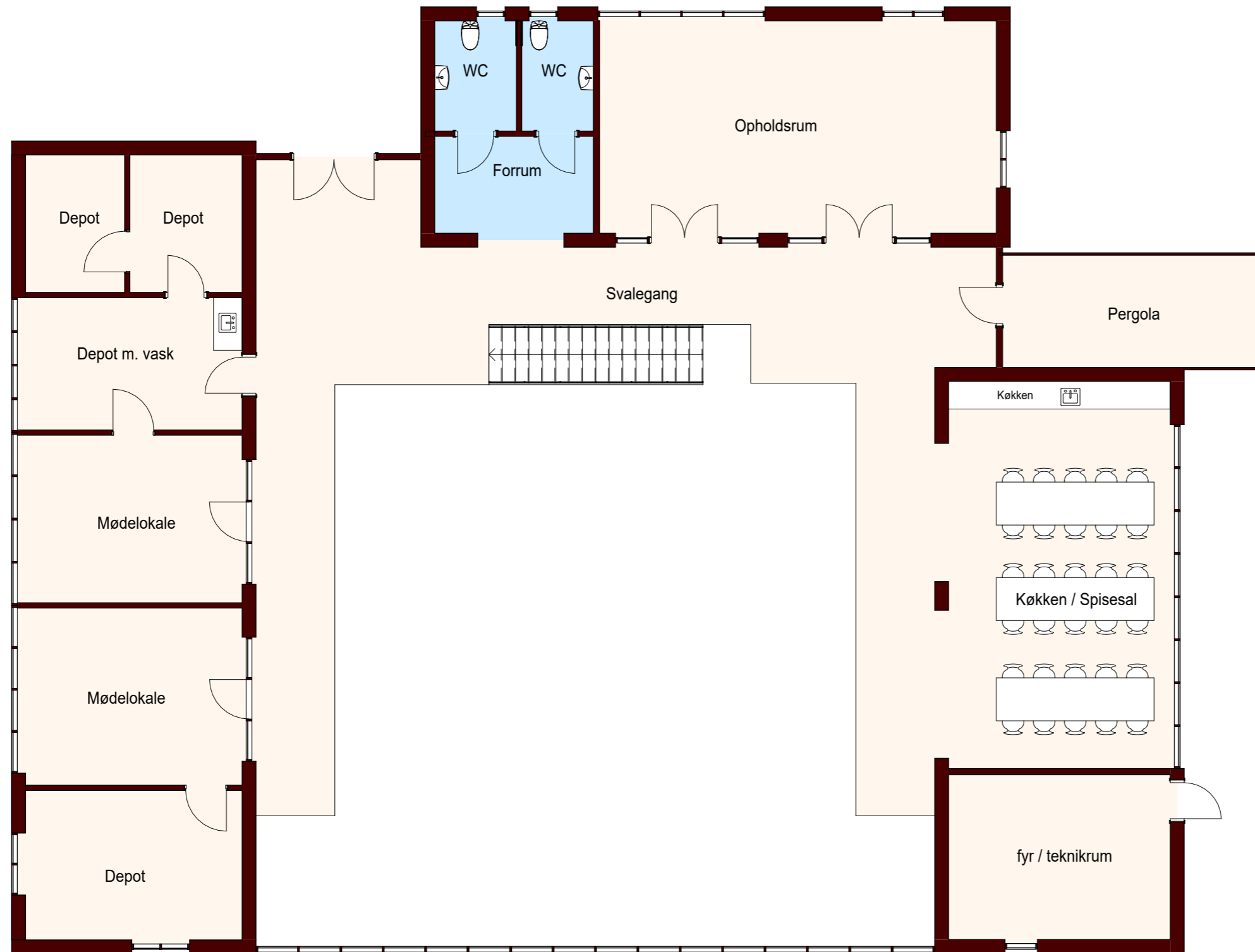
Stueplan Aktivitetshus 1:150
